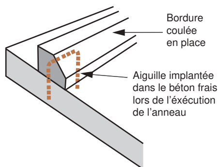
Figure 20 : ancrage de bordure.
