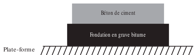
Figure 2b : structure composite constituée d'un revêtement béton à joints non goujonnés posé sur une fondation en grave-bitume.
